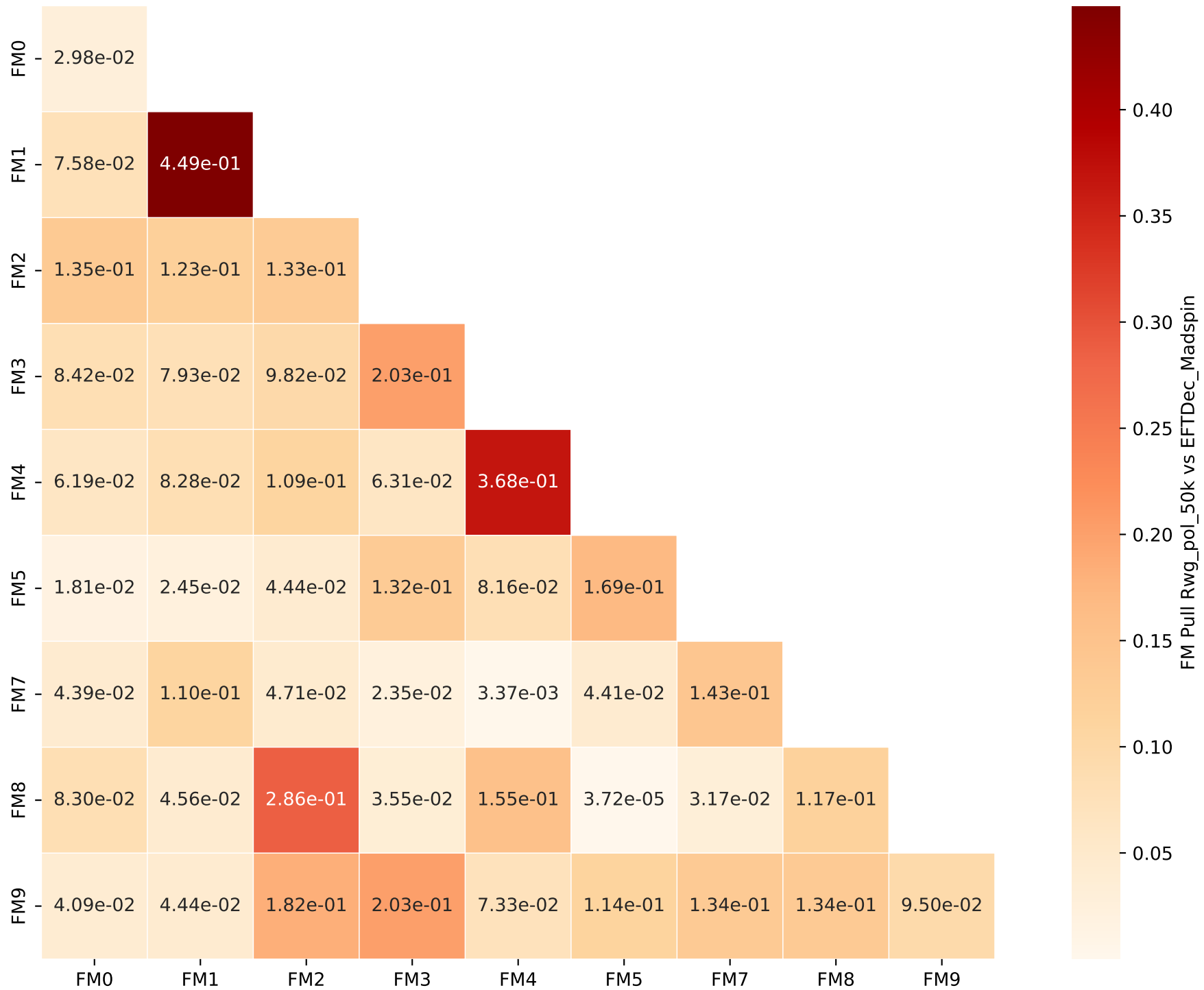
FM Pull Rwg_pol_50k vs EFTDec_Madspin
